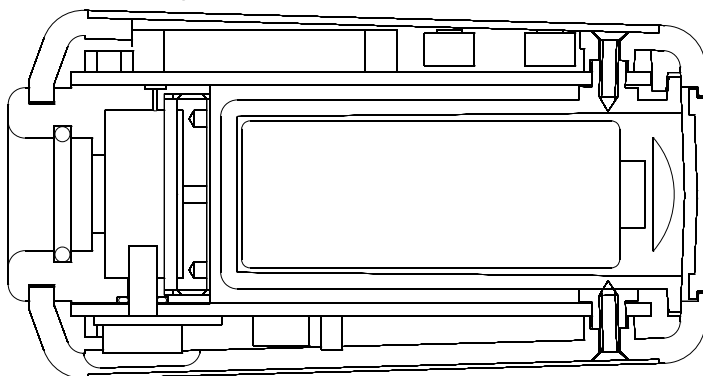
Fig. 3 Construction mécanique du calibre (section).
