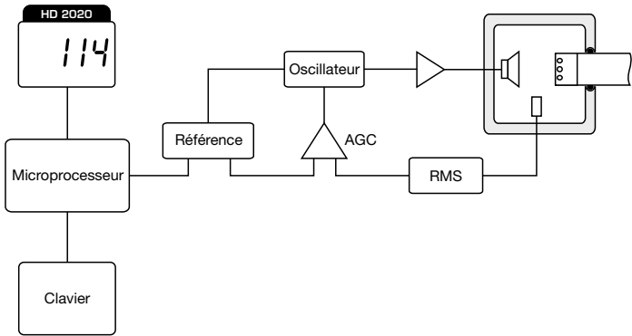
Fig. 4 Schéma de principe de l'électronique.
